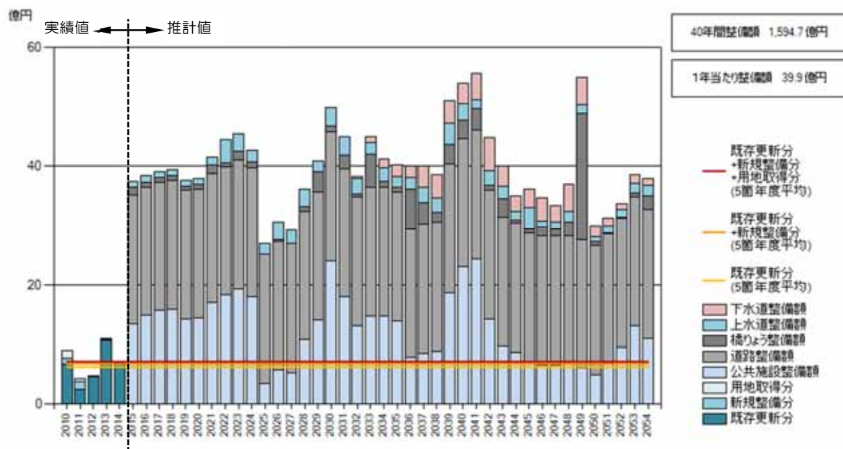
図 1-35 公共施設等全体の更新費用
