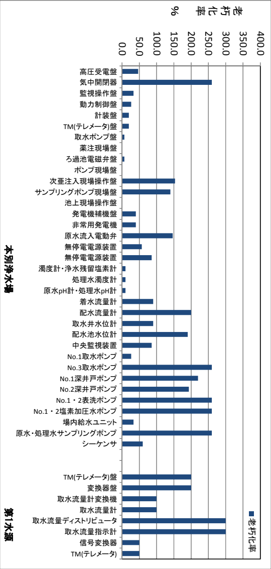
図 4-5 上水道施設の老朽化率
