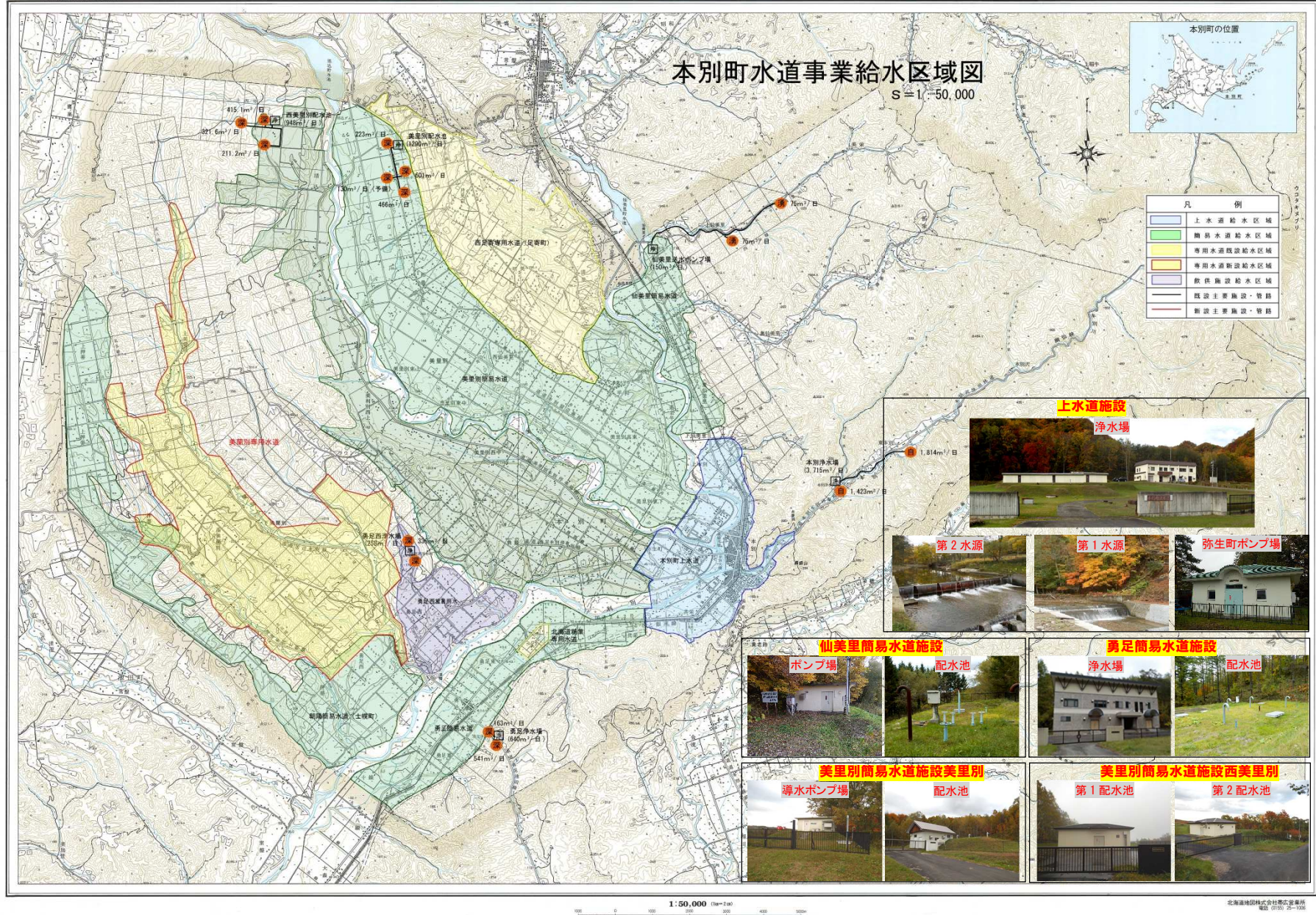
図 2-1 給水区域図
