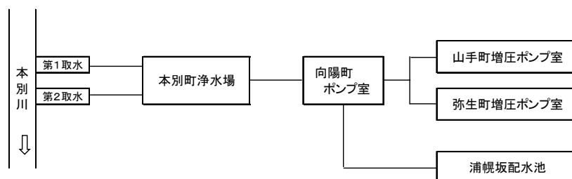
図 2-2 システム図
